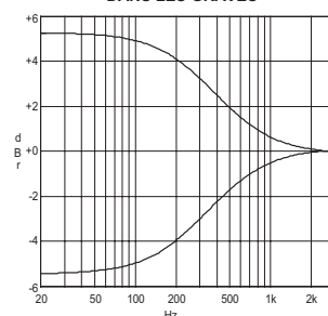
REPONSE EN FREQUENCE DANS LES GRAVES
